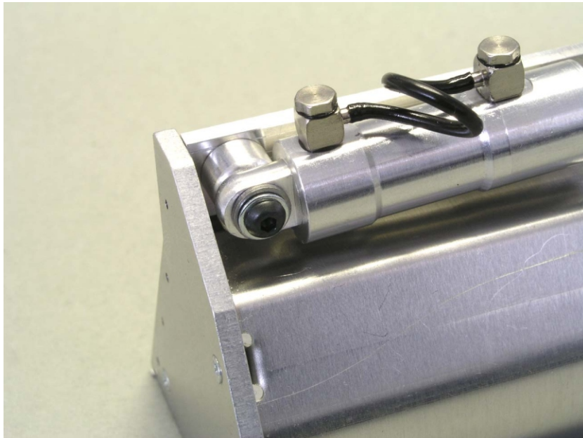
Nebenstehendes Bild zeigt die montierte Schraube .
