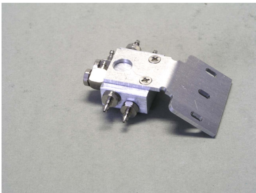
Der Ölverteiler wird mit 2 Schrauben Din 965 M2x4 am kleinen Halteblech angeschraubt .
